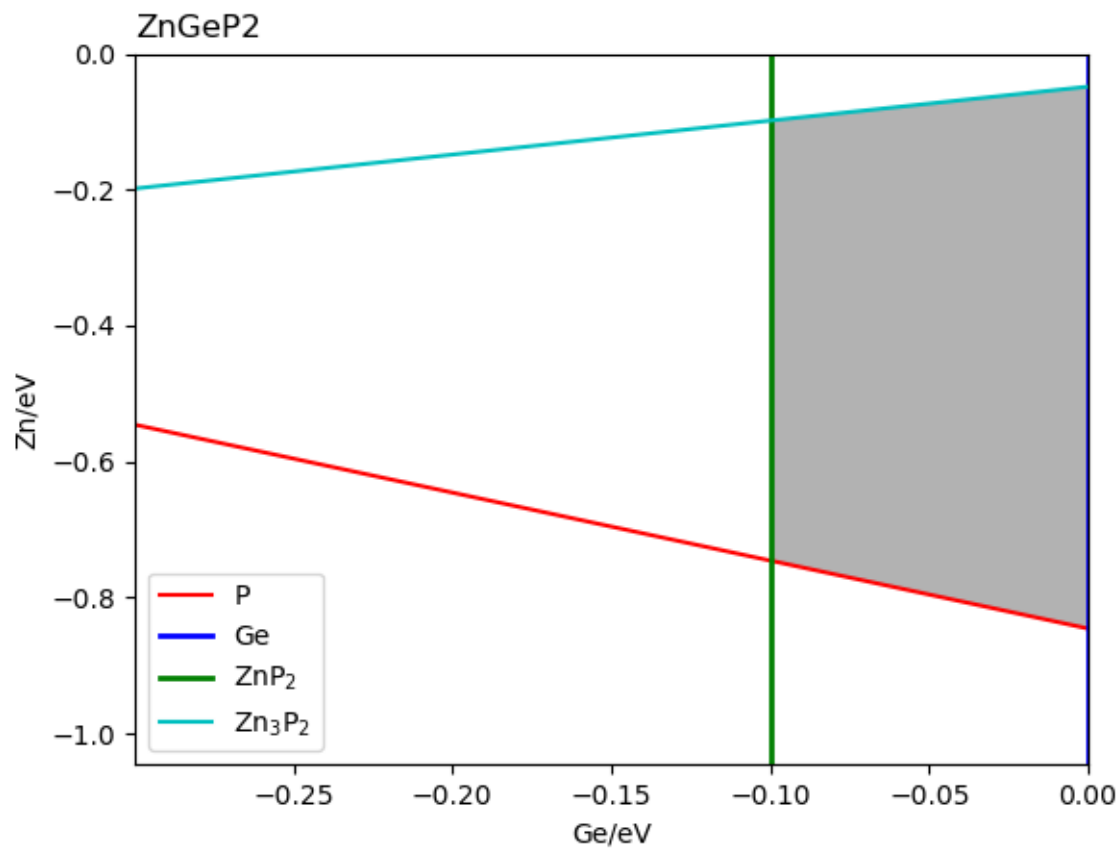
ZnGeP2 的稳定区域图（来自 MP 数据库）。
