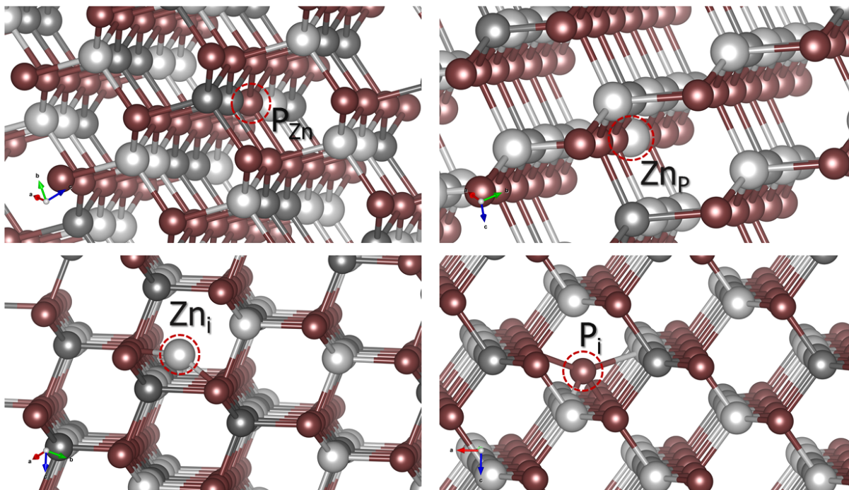
ZnGeP2 超胞部分缺陷结构示意图。
