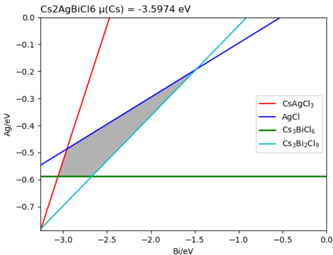
Cs2AgBiCl6 的稳定区域图 (来自第二阶段计算)
