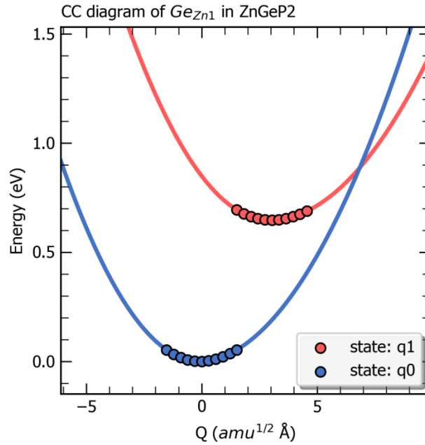
ZnGeP2 中缺陷 \text{Ge}_{\text{Zn1}} 从 +1 价到 0 价的一维位形图。
