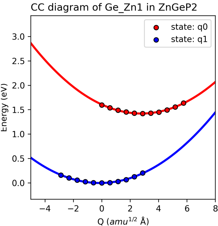
ZnGeP2 中缺陷 Ge_Zn1 的一维位形图。
