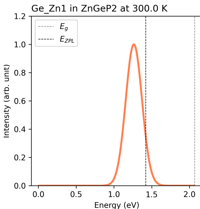
指定温度下 ZnGeP2 中缺陷 Ge_Zn1 的 PL 谱。
