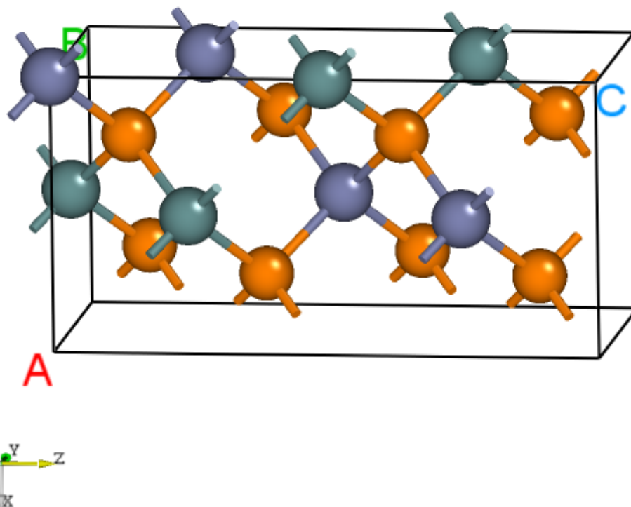
ZnGeP2 的晶体结构。
