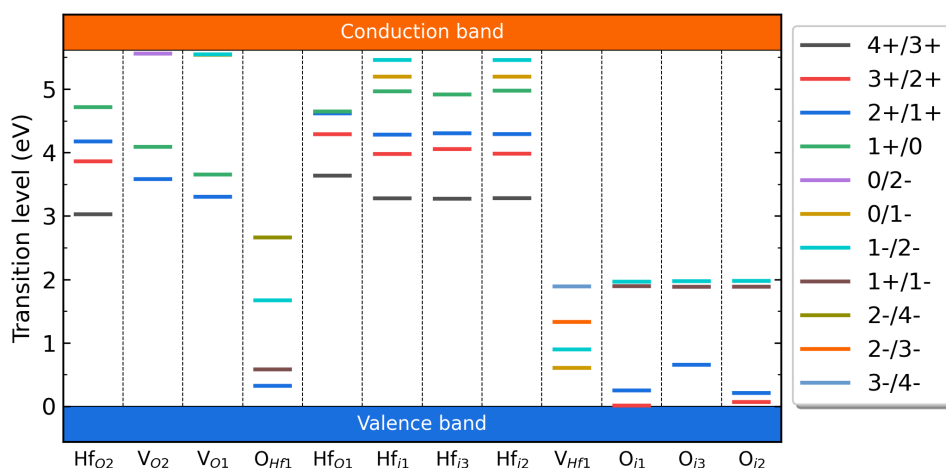
HfO2 各缺陷的转变能级。
