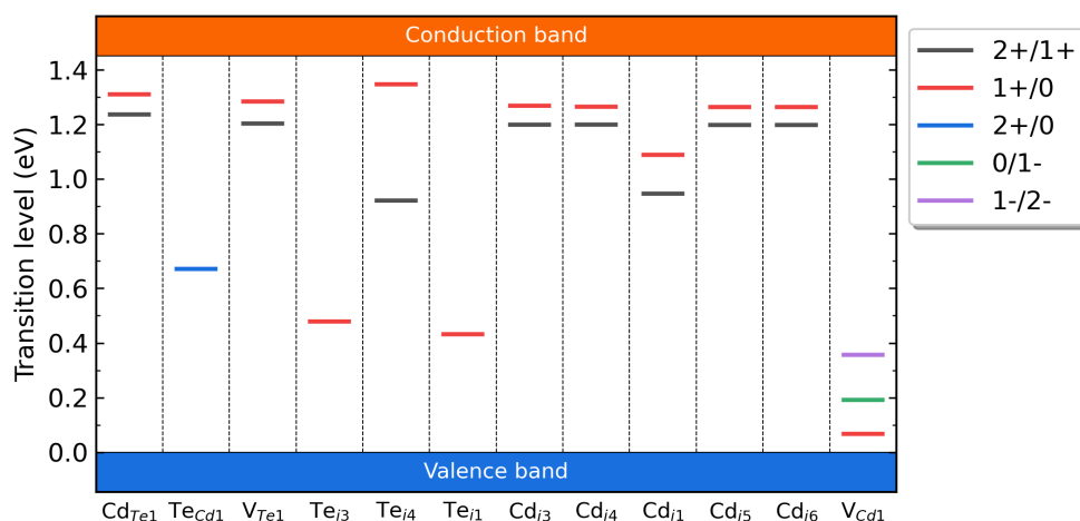
CdTe 的缺陷转变能级。
