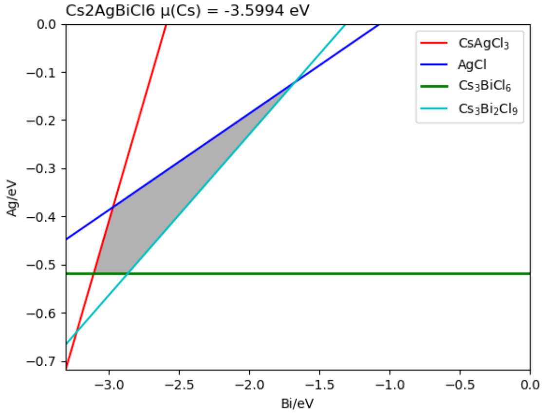
\text{Cs}_2\text{AgBiCl}_6 的稳定区域图（来自 MP 数据库）
