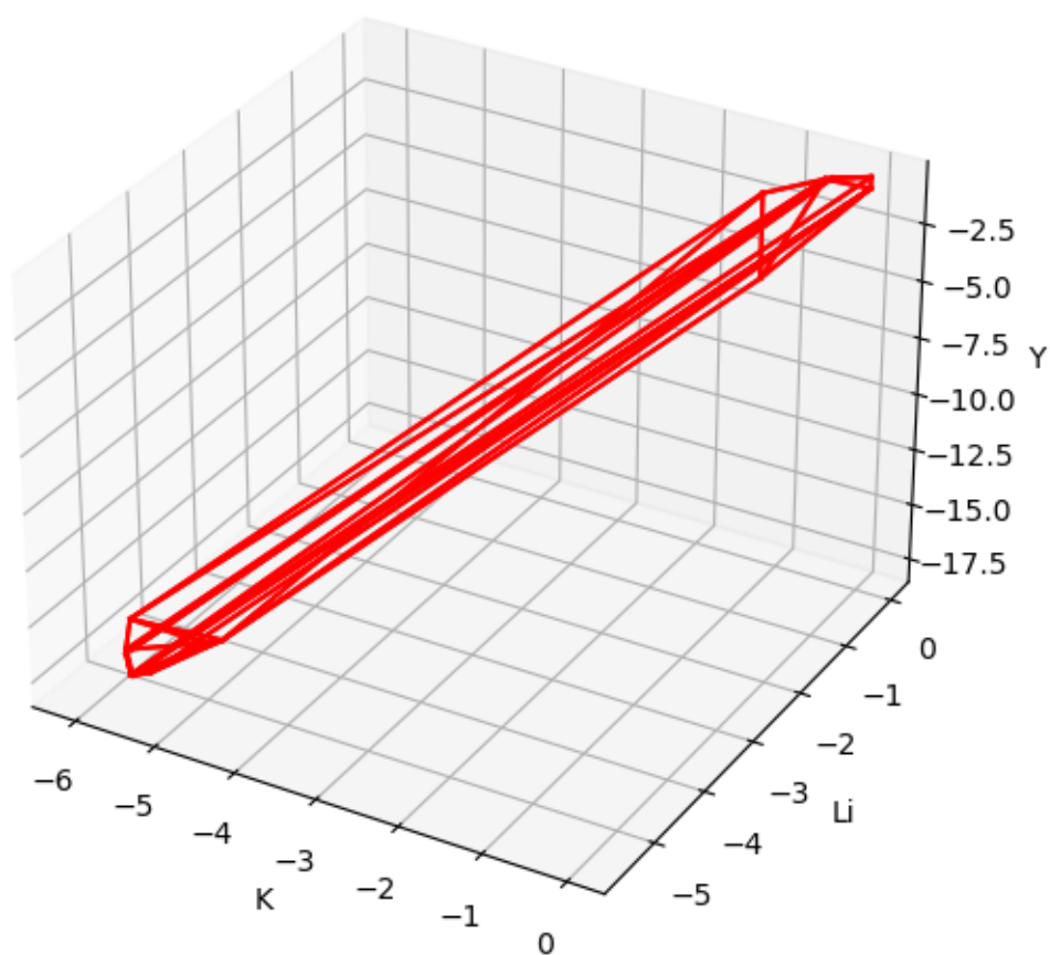
K 2 LiYF 6 的三维稳定区域图（来自第二阶段计算）
