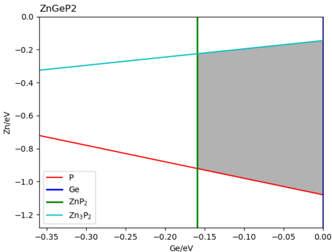
ZnGeP2 的稳定区域图（来自 DFT 计算）。
