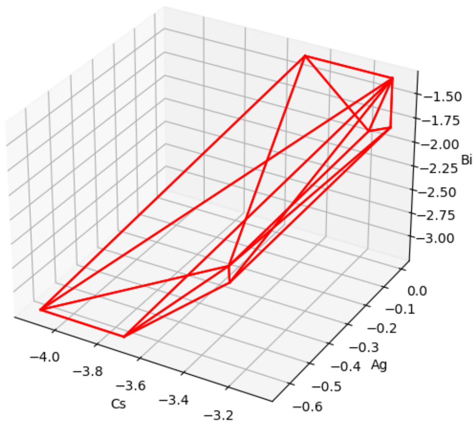
Cs 2 AgBiCl 6 的三维稳定区域图 (来自 MP 数据库)
