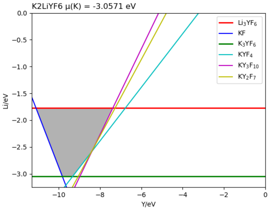
K2LiYF6 的稳定区域图（来自第二阶段分析）
