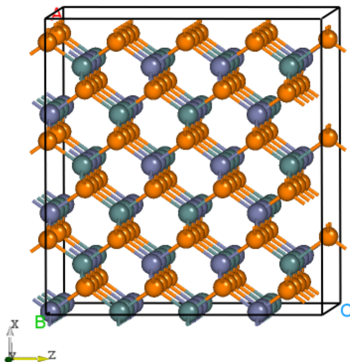
ZnGeP2 的超胞结构。
