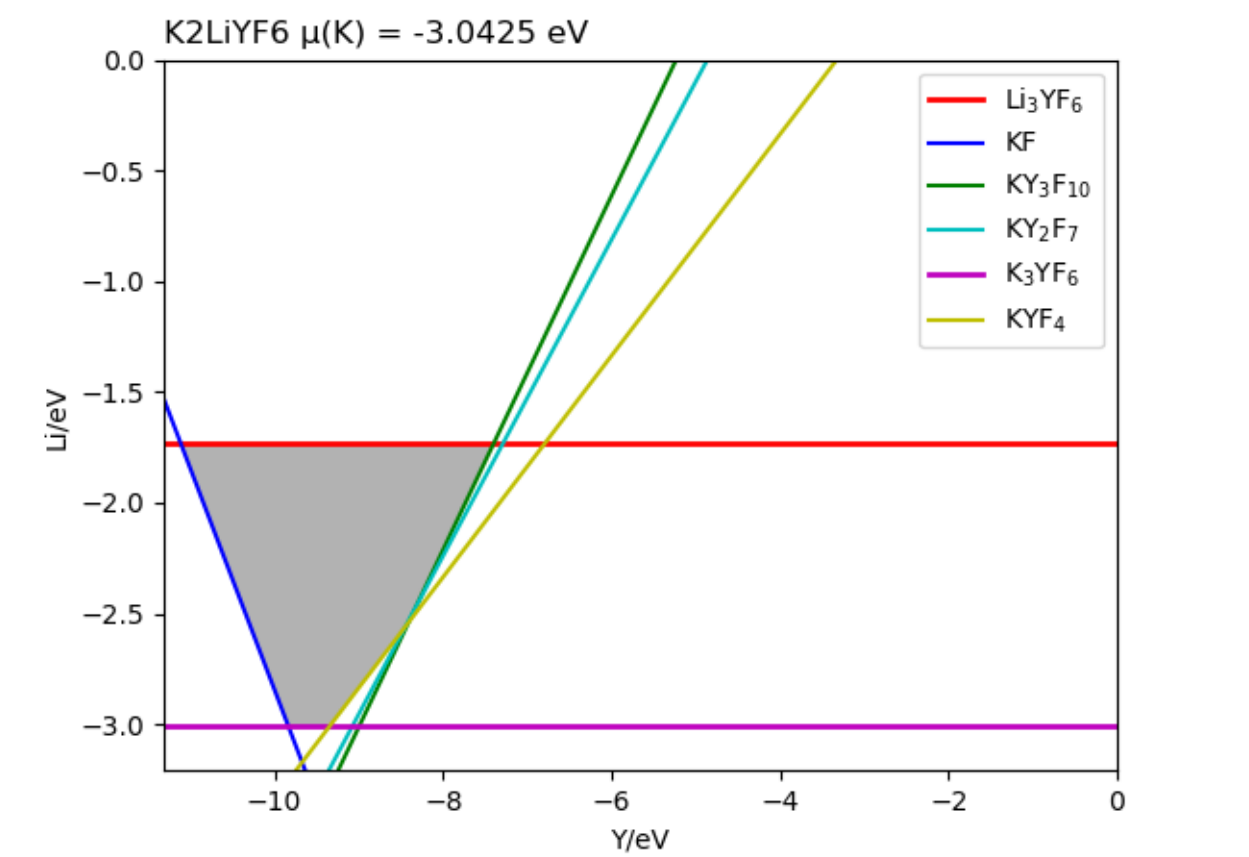
K2LiYF6 的稳定区域图（来自 MP 数据库）
