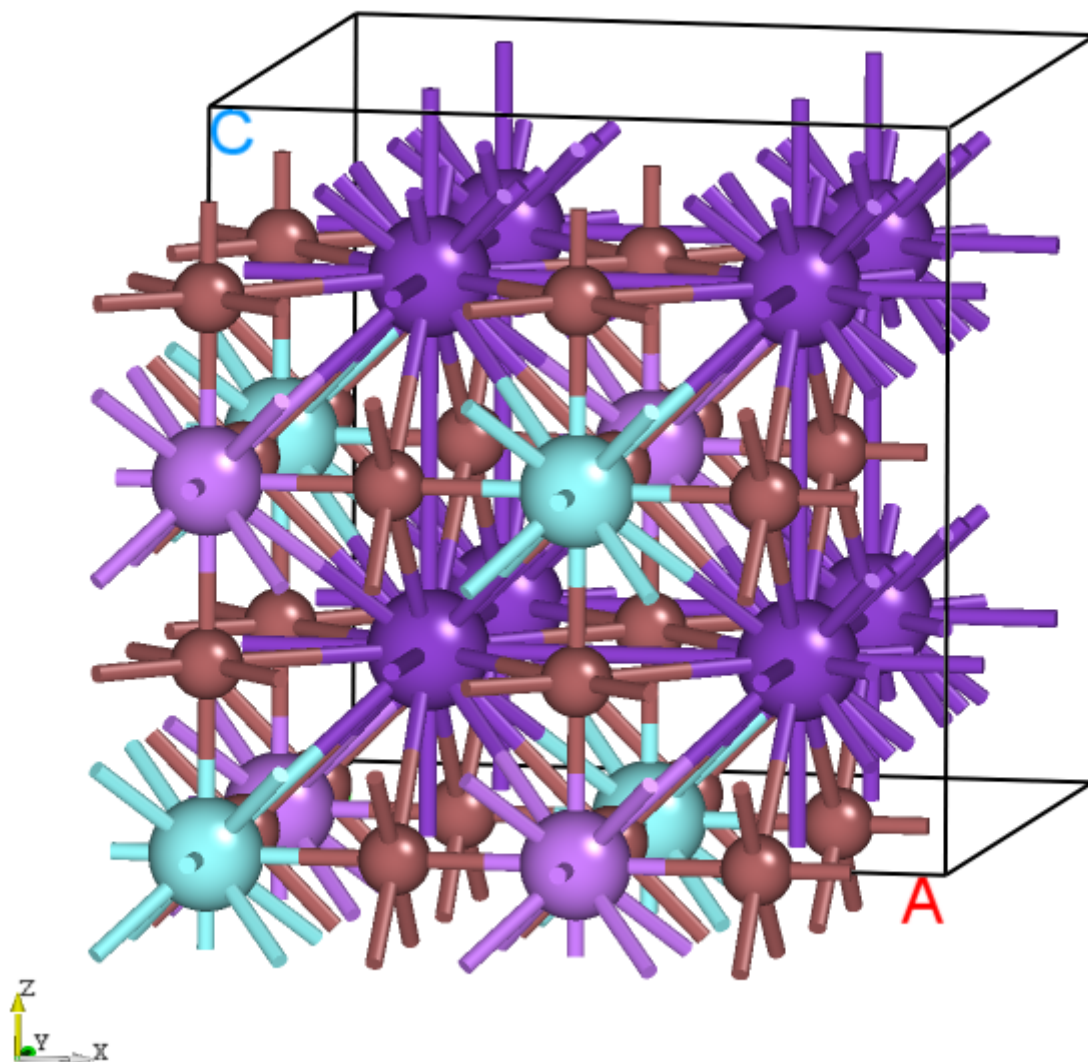
K 2 LiYF 6 的晶体结构示意图
