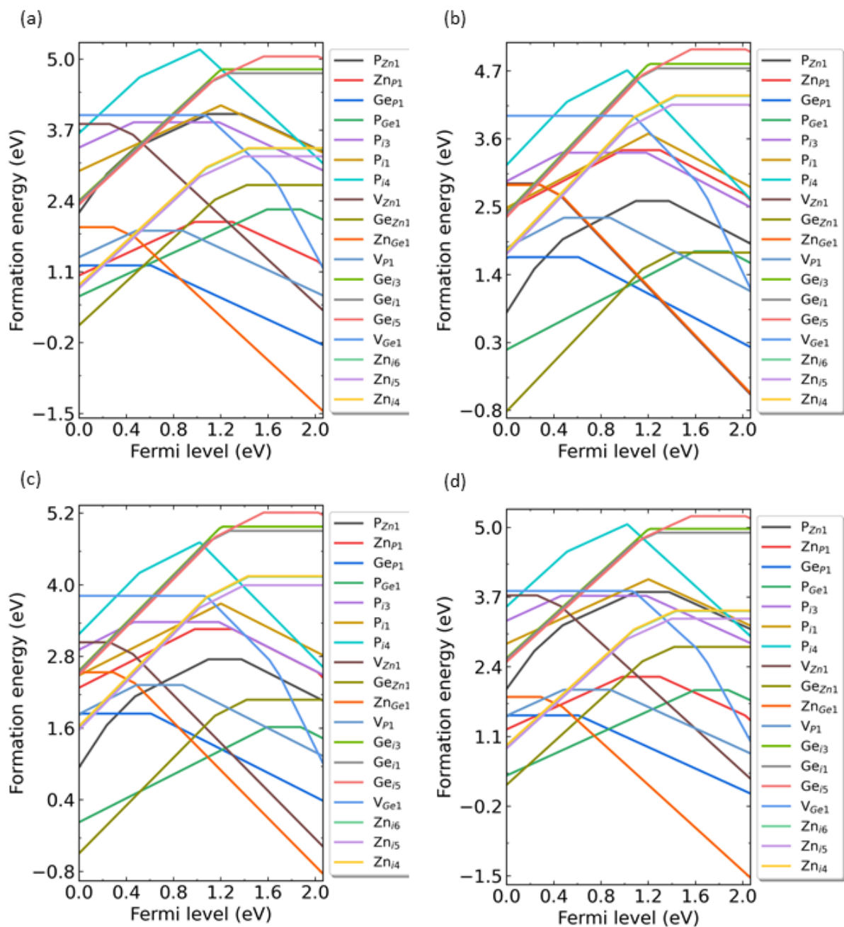
ZnGeP 2 各类缺陷在化学势点 (a) p1, (b) p2, (c) p3, (d) p4 处的形成能随费米能级的变化。
