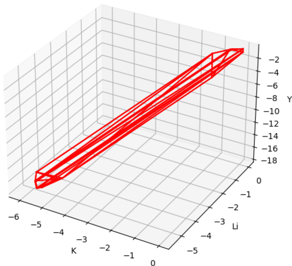
K2LiYF6 的三维稳定区域图 (来自 MP 数据库)
