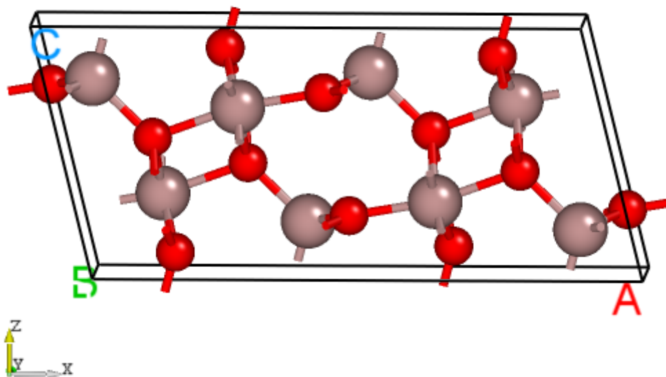
Ga 2 O 3 的晶体结构。
