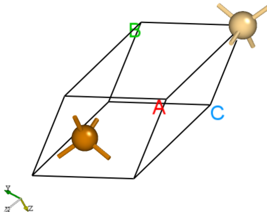
CdTe 的原胞结构。
