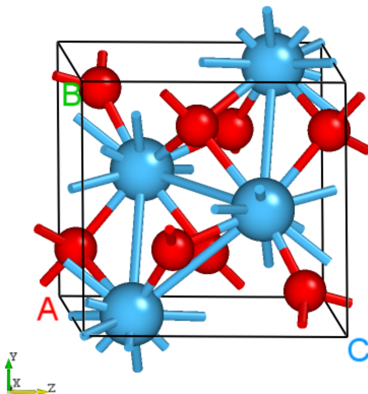
HfO 2 的晶体结构。
