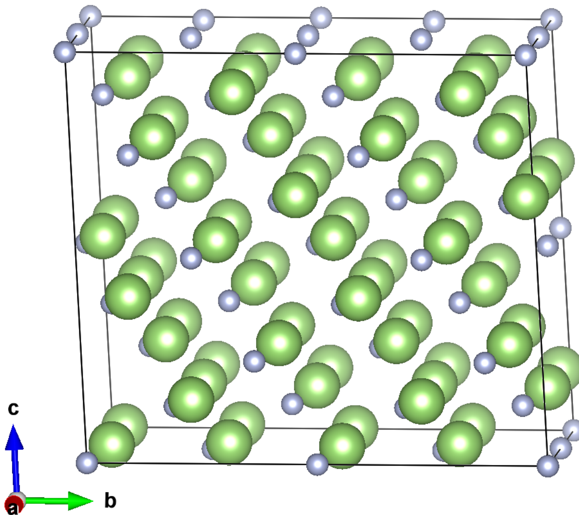
GaN 的超胞结构。
