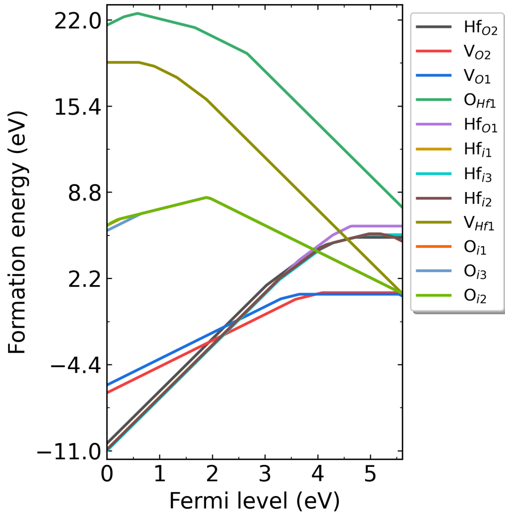
HfO 2 在 p1 处 (Hf-rich) 的缺陷形成能随费米能级的变化。
