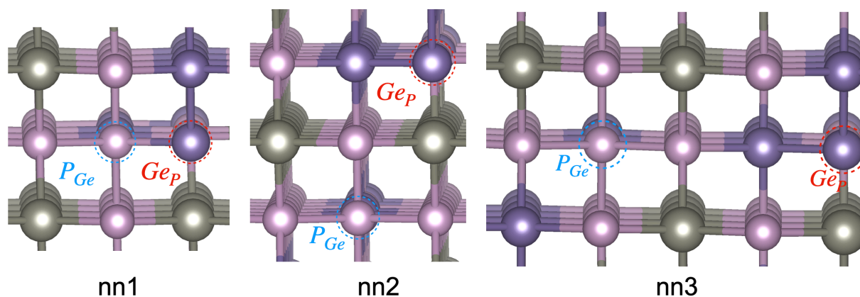
DASP 产生的三种 Ge_{P1} + P_{Ge1} 复合缺陷构型。
