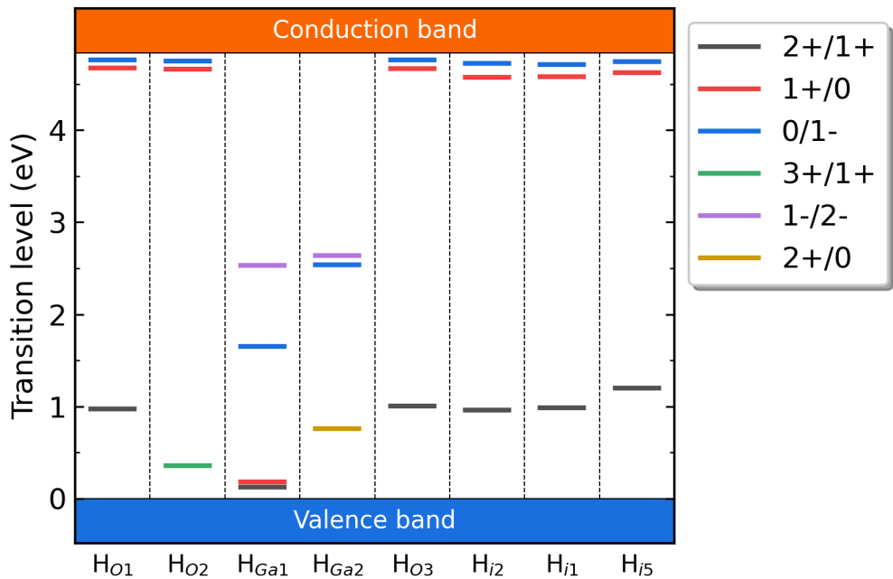
掺杂 H 的 Ga2O3 各缺陷的转变能级。
